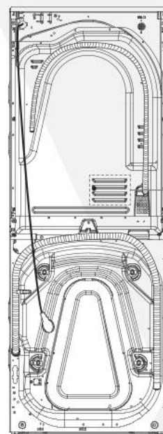
Visão traseira
